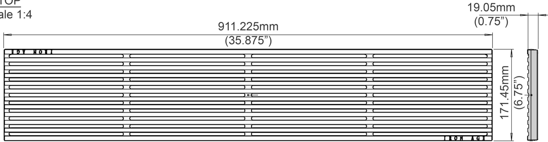
EDGE scale 1:4
